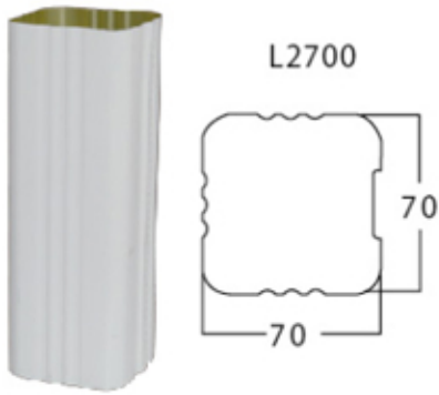
たて樋型
