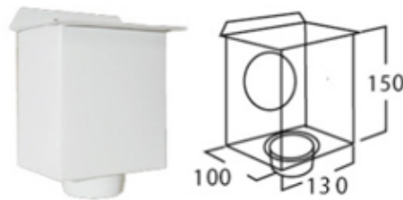
箱マス
